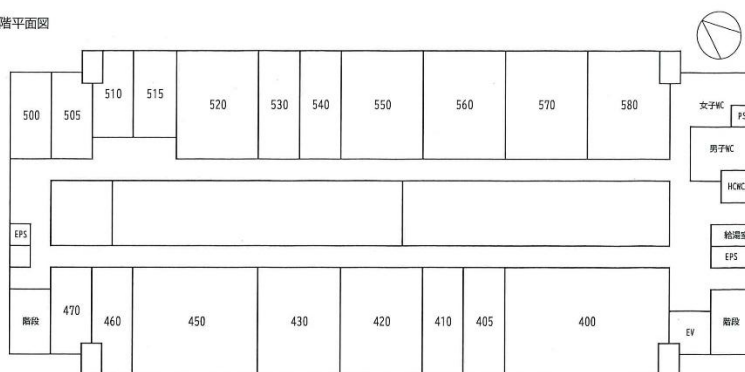
3階平面図
